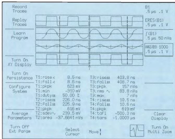
Automatic pulse parameter readout in a 7200A.
